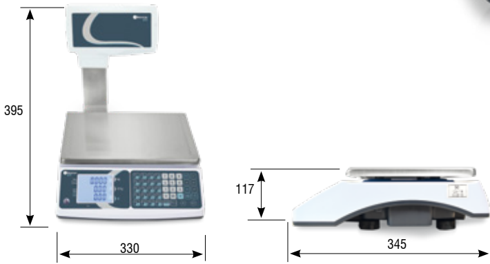
Dimensioner (mm)
